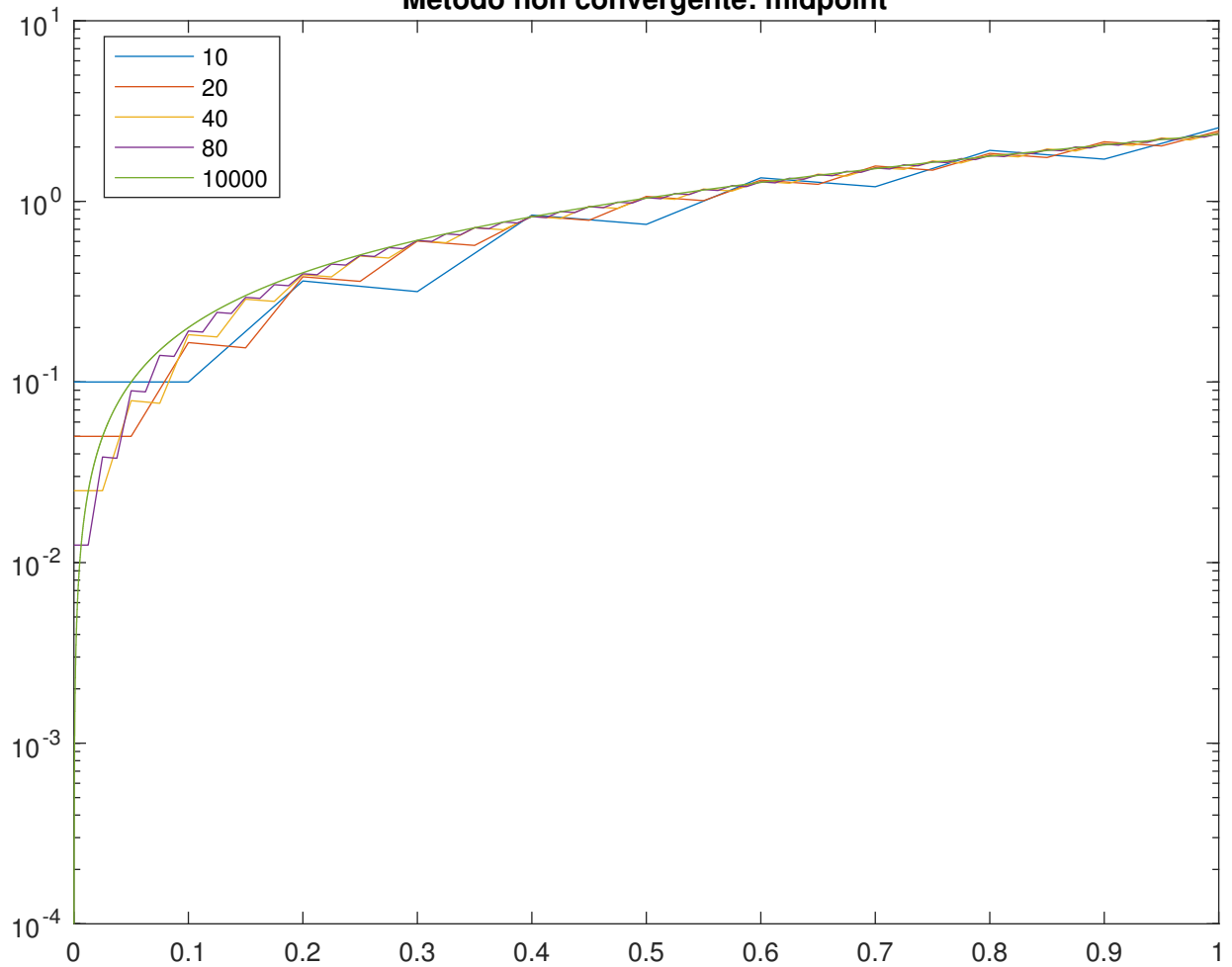
Metodo non convergente: midpoint
