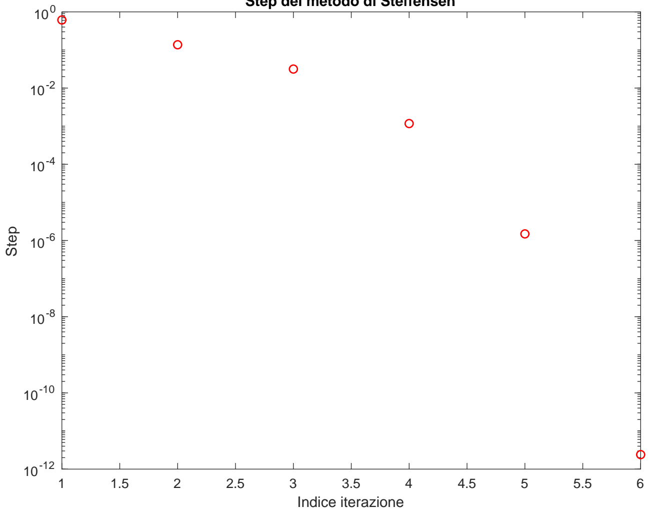
Step del metodo di Steffensen
