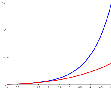
Figura: Grafico della funzione f(x) = \exp(x) (in blu ), p(x) = 1 + x + \frac{x^2}{2} + \frac{x^3}{6} (in rosso ), nell'intervallo [0, 5] .
