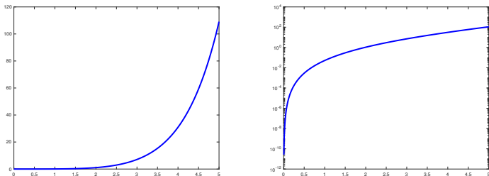
Figura: Differenza tra plot e semilogy nel rappresentare i grafici unendo mediante un segmento le coppie (x_k, |f(x_k) - p(x_k)|) per t = 1, \dots, 1000 .
