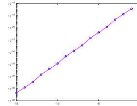
Figura 7: Grafico della funzione \text{eps}(x) per x \in [10^{-15}, 10^{-1}] , mostrando i valori assunti in 10^{-15}, 10^{-14}, \dots, 10^{-1} .
