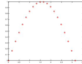
Figura 4: Grafico delle coordinate (x_k, \sin(x_k)) , per x_k = 0 + (k-1)\pi/19 , k = 1, \dots, 20 .
