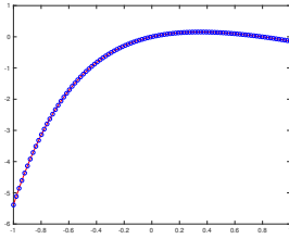
Figura 8: Grafico della funzione f(x) = 1 - x - \exp(-2x) per x \in [-1, 1] (in rosso), con cerchietti blu in (x_k, f(x_k)) , x_k = -1 + 2(k-1)/49 , k = 1, \dots, 50 .
