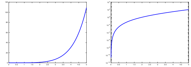
Figura 3: Differenza tra plot e semilogy nel rappresentare le coppie (x_k, |f(x_k) - p(x_k)|) per t = 1, \dots, 1000 .
