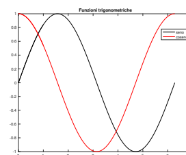
Figura 5: Grafico di \sin(x) , \cos(x) in [0, 2\pi] , con titolo e legenda.
