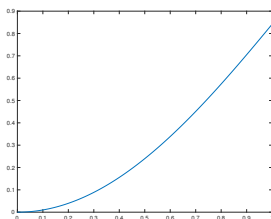
Figura 1: Grafico della funzione f(x) = x \cdot \sin(x) , nell'intervallo [0, 1] .
