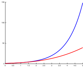
Figura 2: Grafico della funzione f(x) = \exp(x) (in blu), p(x) = 1 + x + \frac{x^2}{2} + \frac{x^3}{6} (in rosso), nell'intervallo [0, 5] .
