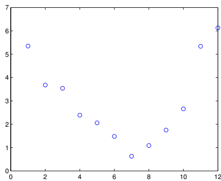
Figura 6: Grafico di alcuni dati immagazzinati su file.
