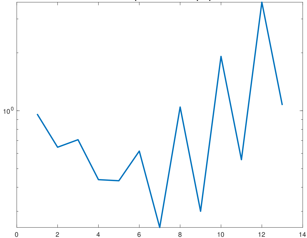
Errori di interpolazione: nodi equispaziati
