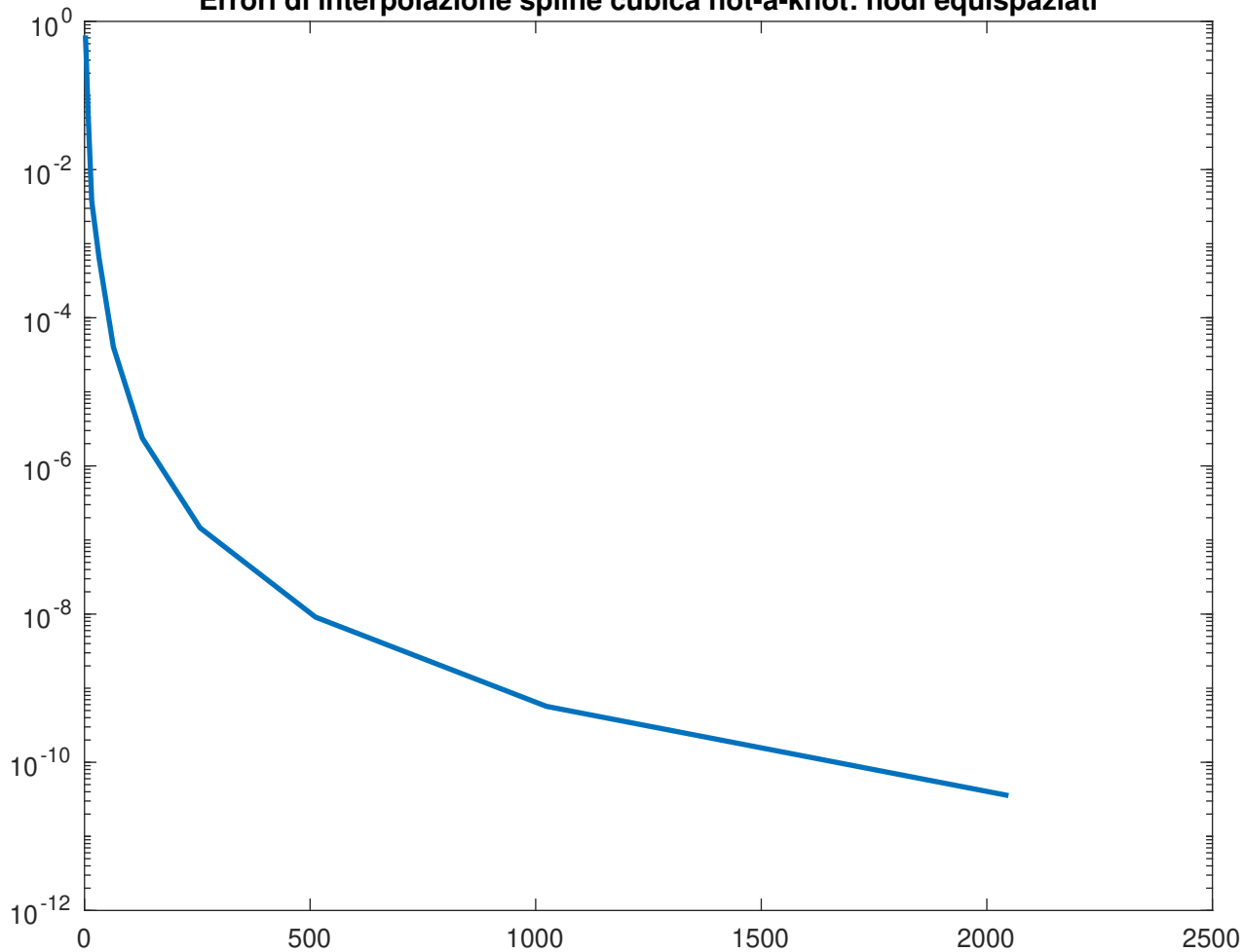
Errori di interpolazione spline cubica not-a-knot: nodi equispaziati
