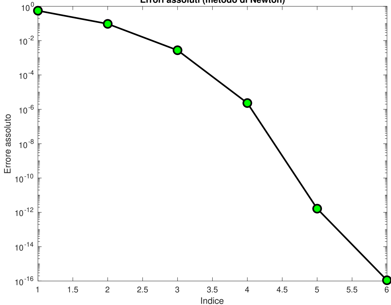
Errori assoluti (metodo di Newton)
