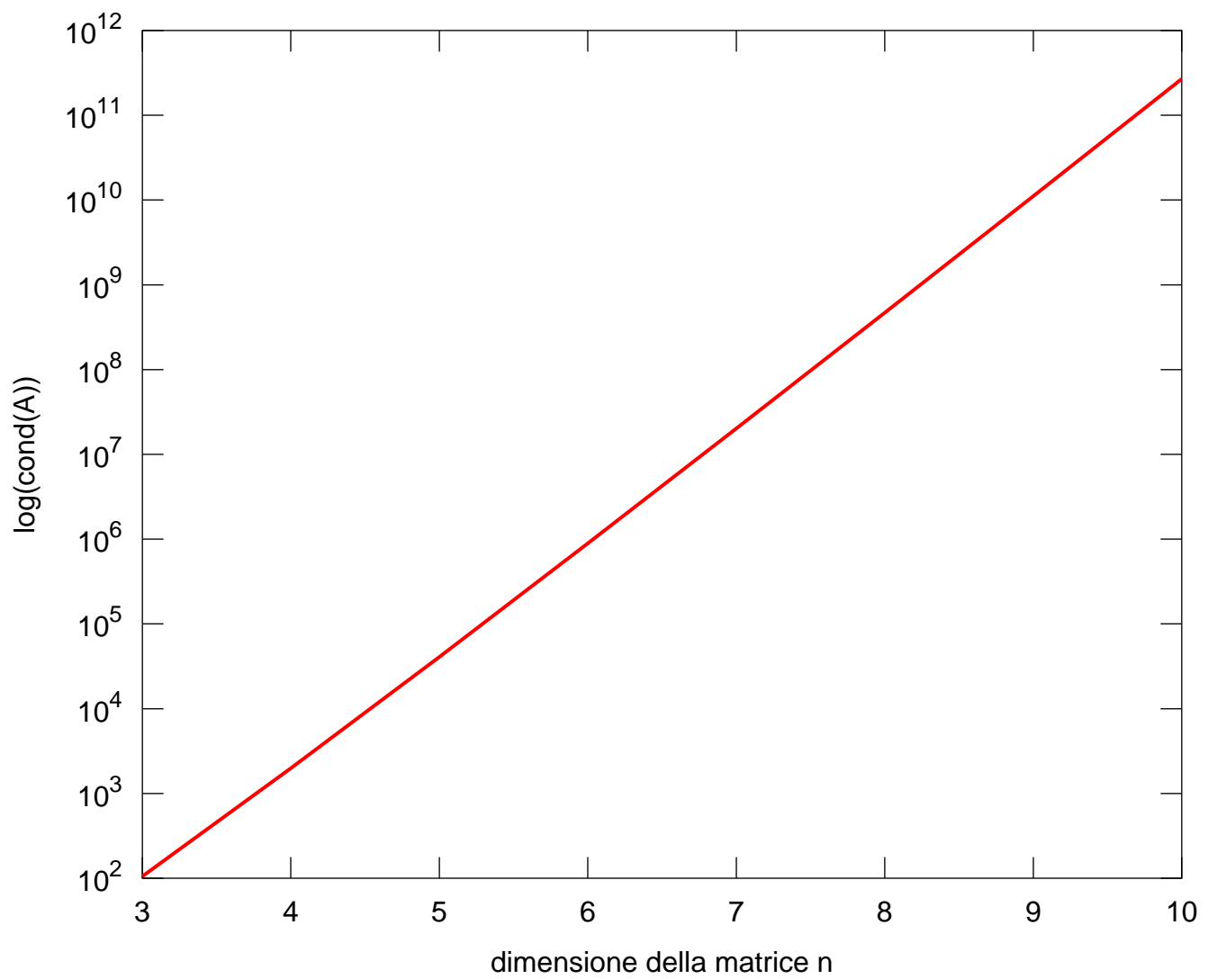
Condizionamento della matrice di Vandermonde
