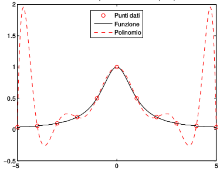
Polinomio interpolante e funzione 1/(1+x.^2)
