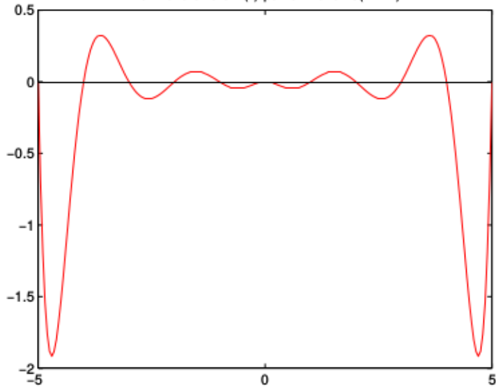
Funzione errore E(x) per funzione 1/(1+x^2)
