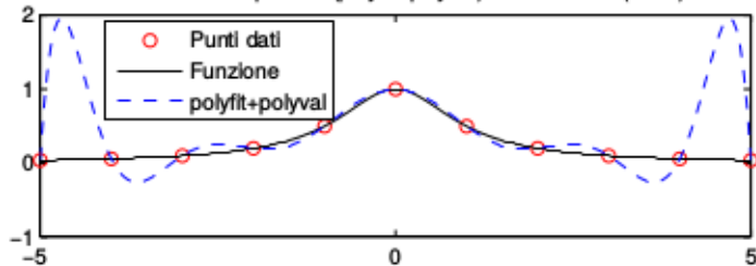
Polinomio interpolante (polyfit+polyval) e funzione 1./(1+x.^2)
