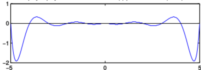
polyfit+polyval - Funzione errore E(x) per funzione 1./(1+x.^2)
