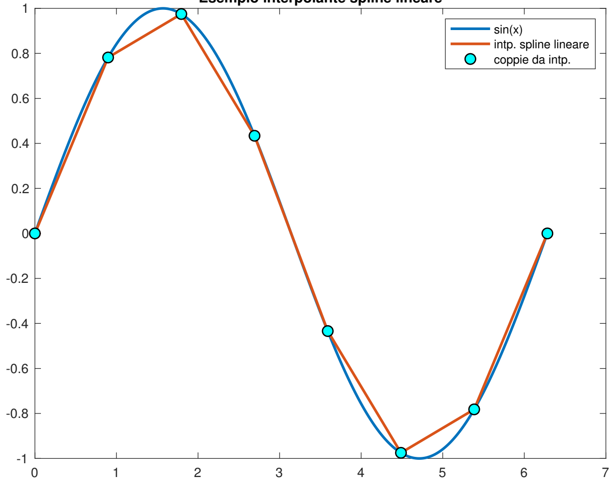
Esempio interpolante spline lineare
