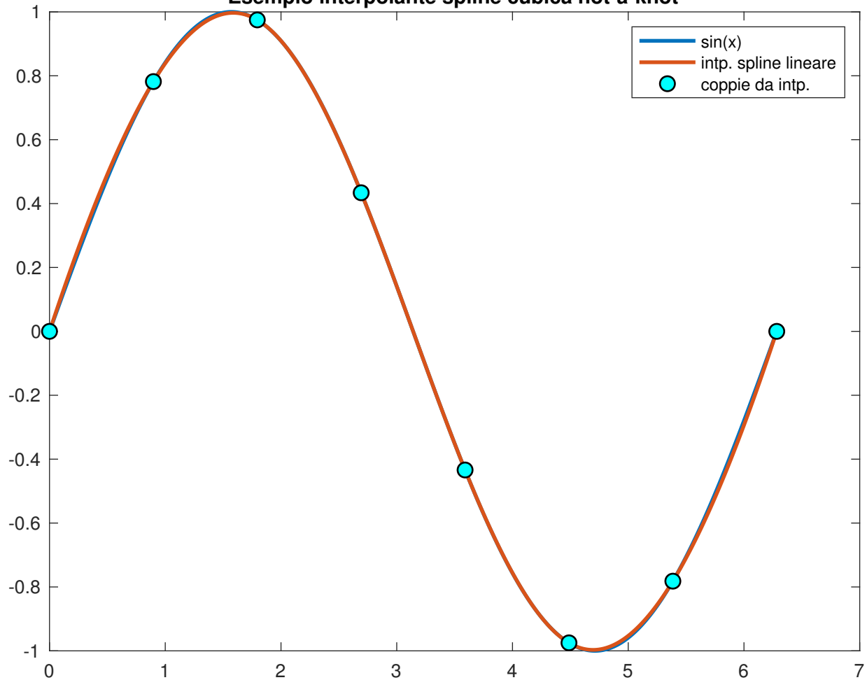
Esempio interpolante spline cubica not-a-knot
