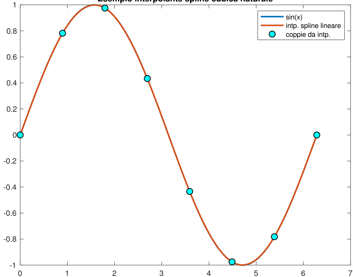
Esempio interpolante spline cubica naturale
