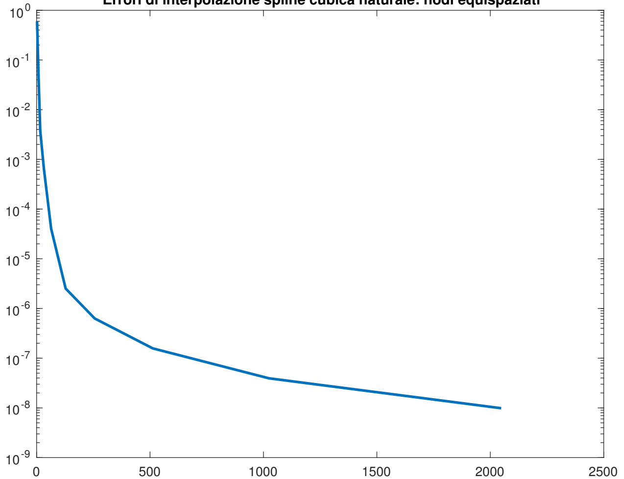
Errori di interpolazione spline cubica naturale: nodi equispaziati
