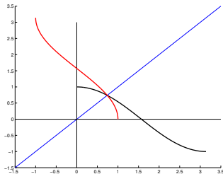
Figura : La funzione f(x) = \cos(x) in [0, \pi] (nero), f^{-1}(y) = \arccos y
