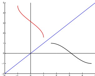
Figura : La funzione f(x) = \sin(x) in [\pi/2, 3\pi/2] (nero), f^{-1}(y) (rosso).
