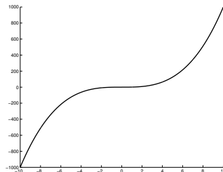
Figura : La funzione f(x) = x^3 in [-10, 10] .
