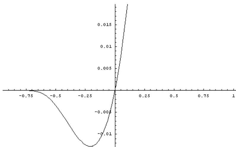
Figura 5: Esercizio 1.4 (nell'intorno dello 0)
