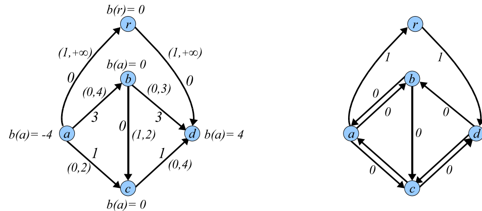
(a) Trovato flusso ammissibile per D (il flusso di partenza in Figura 1(a)).
