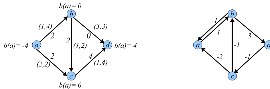
Figura 1: Esecuzione dell'algoritmo di cycle canceling: la colonna a sinistra rappresenta il grafo originale con il flusso ad ogni iterazione, quella a destra rappresenta il grafo residuo relativo al flusso corrente, con i costi c' sugli archi.
