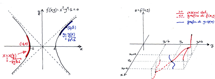
(a) Funzioni implicite definite da f(x, y) = x^2 - y^2 - 1 = 0 . (b) L'idea della dimostrazione del Teorema del Dini nel caso base.
