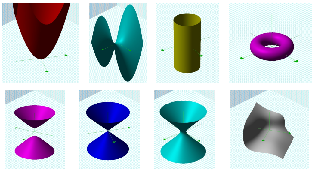
Esempi di superfici in \mathbb{R}^3 . (a-b) Paraboloide ellittico ed iperbolico. (c) Cilindro. (d) Toro. (e-f-g) Il luogo z^2 - x^2 - y^2 = \alpha è un iperboloide a una/due falde se \alpha \leq 0 ; un cono bilatero se \alpha = 0 . (h) La superficie x^3 + 2y^3 + 4z^3 - xy + 4 = 0 dell'esercizio.
