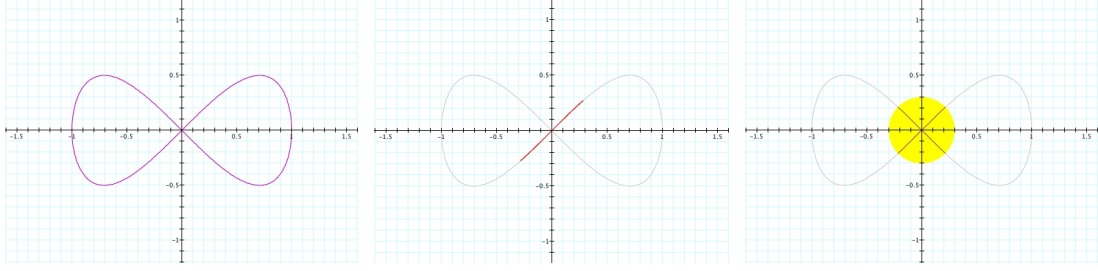
(a) Il sostegno della curva otto. (b) Il segmento ]-\frac{\pi}{11}, \frac{\pi}{11}[ \subset \mathbb{R} , intorno di t_0 = 0 , è diffeomorfo alla sua immagine \gamma(]-\frac{\pi}{11}, \frac{\pi}{11}[) \subset \mathbb{R}^2 , che è il tratto di curva otto evidenziato in rosso: il Teorema delle Immersioni è rispettato. (c) La “ics” porpora che l’intorno giallo di (0, 0) in \mathbb{R}^2 individua sulla curva otto non può essere diffeomorfo ad un intervallo di \mathbb{R} .
