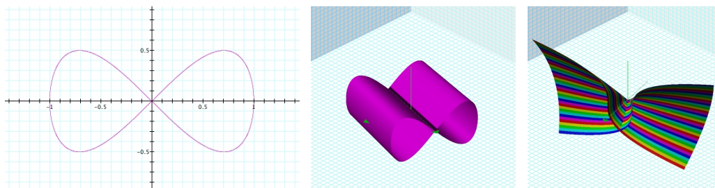
(a) La curva otto, che (b), traslata, dà luogo a una superficie parametrica singolare. (c) Un’altra superficie parametrica singolare.
