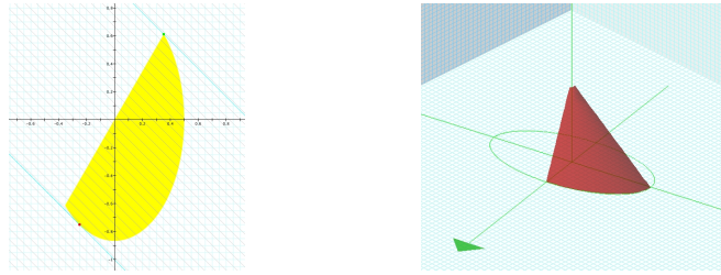
(a) Il compatto D e le curve di livello di f(x, y) = x + y . (b) La porzione di cono pieno X .
