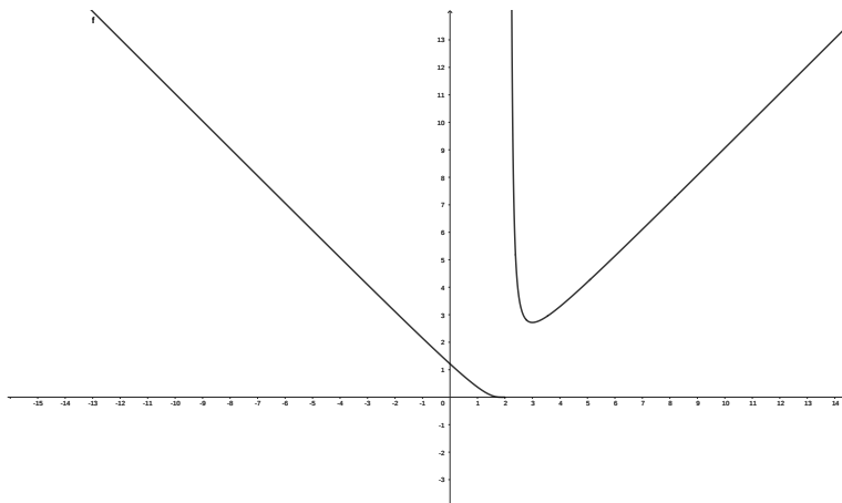
Figure 1: abbozzo del grafico della funzione dell'esercizio 1.
