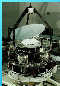
Sonda Giotto
