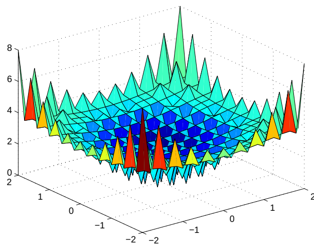
Figura 9: Interpolazione RBF con multiquadratica inversa e \epsilon = 10^{-2} .
