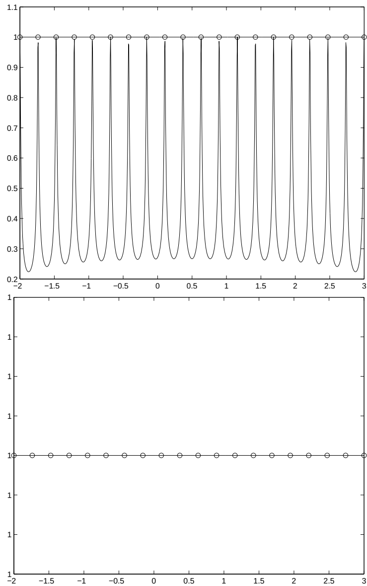
Figura 2: Funzione costante.
