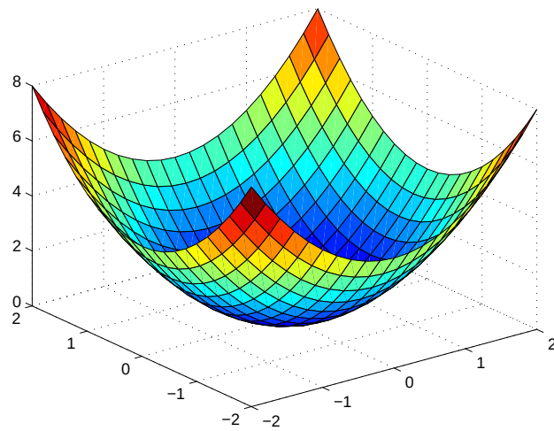
Figura 8: Interpolazione RBF con multiquadratica inversa e \epsilon = 10^{-1} .
