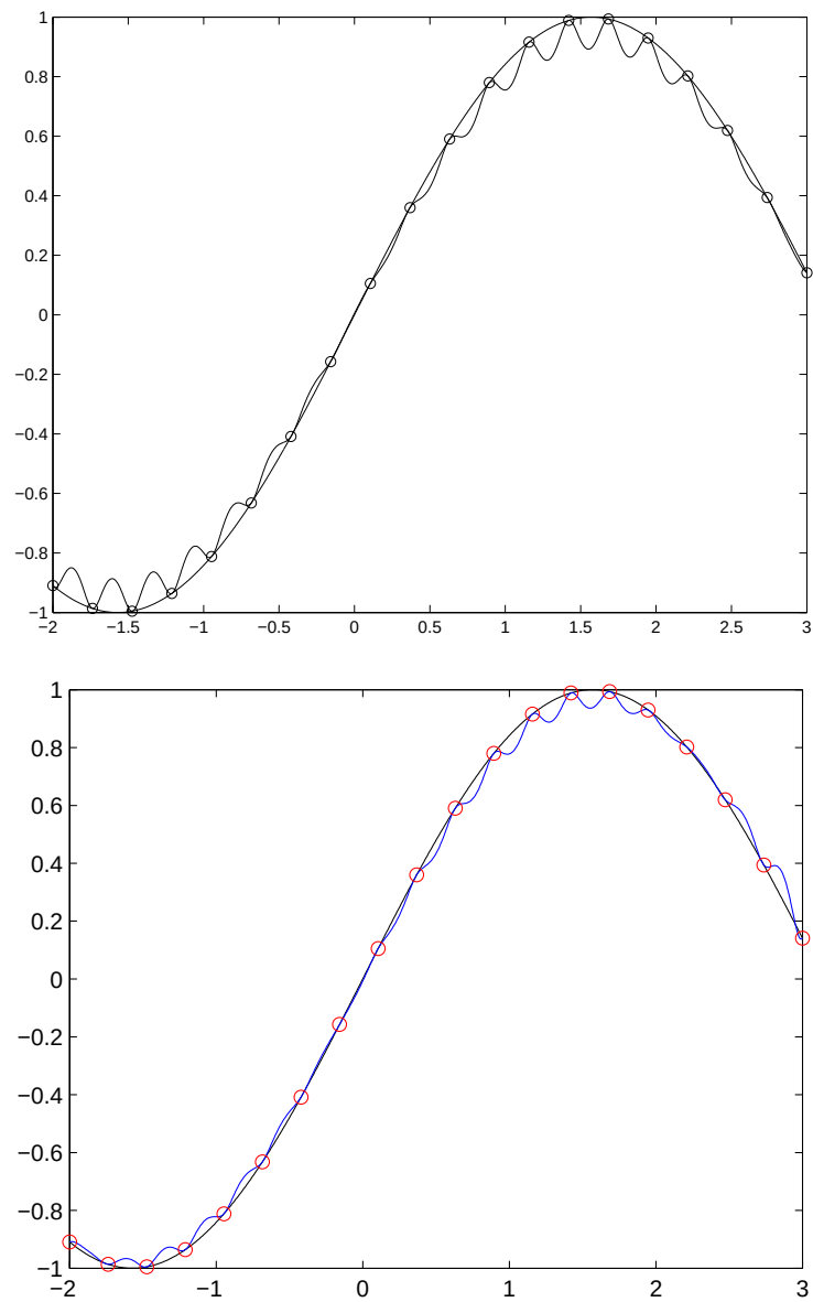
Figura 4: Funzione \sin .
