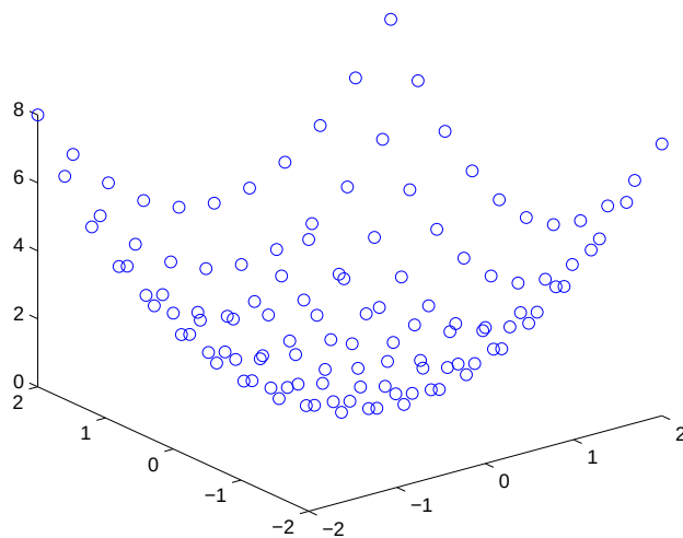
Figura 7: Punti di interpolazione
