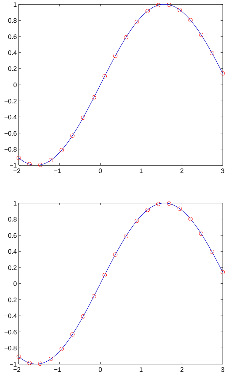
Figura 5: Funzione \sin .
