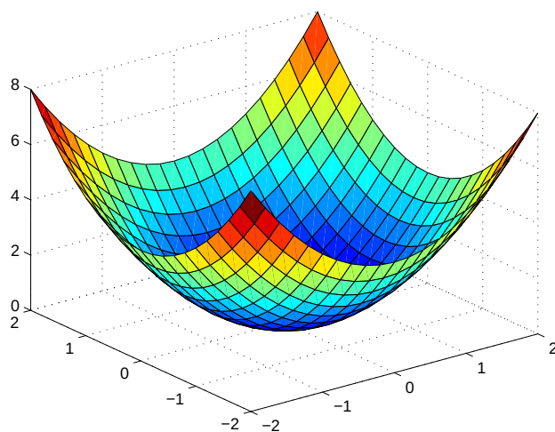
Figura 6: Funzione originaria
