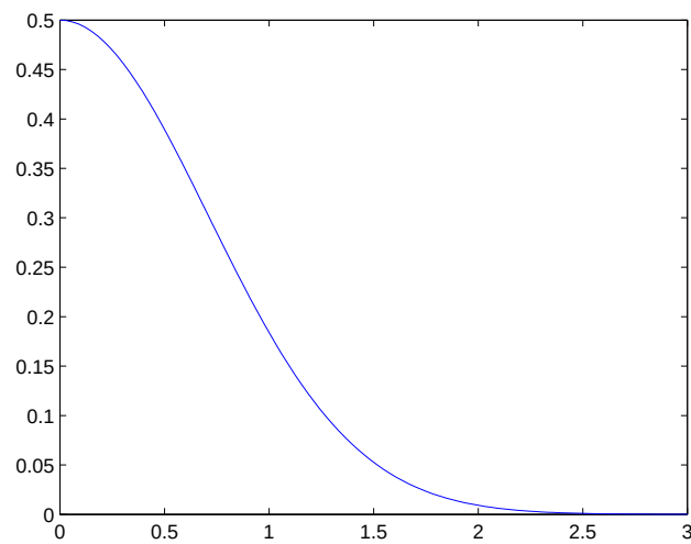
Figura 1: Esempio di funzione base gaussiana.
