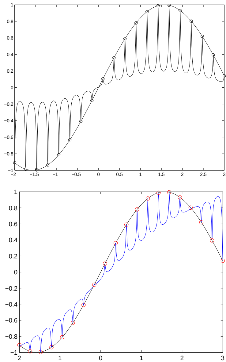
Figura 3: Funzione \sin .
